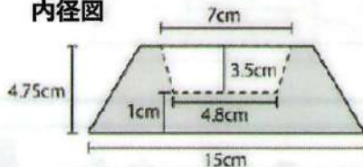
内径図
