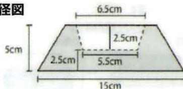
内径図
